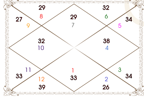
ஸர்வாஜ்டகவர்க்க
