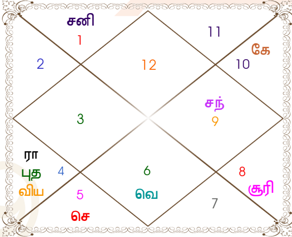
நவாமிச அட்டவணை
